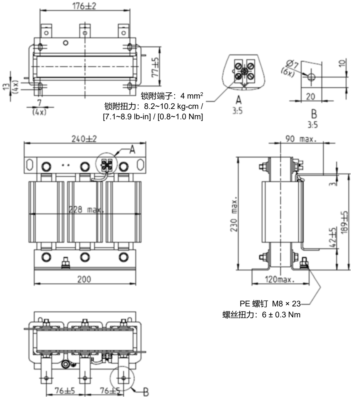
图 7-13 单位: mm
