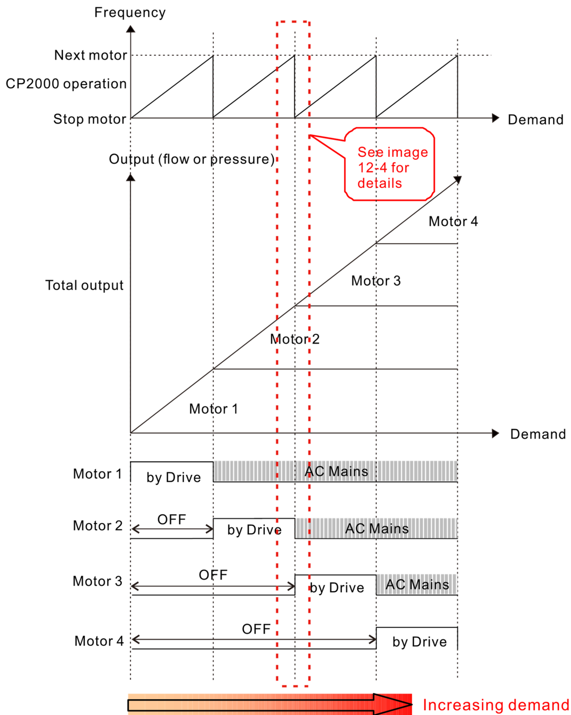
图 12-3 PID 定量循环动作时序 – 增加需求
