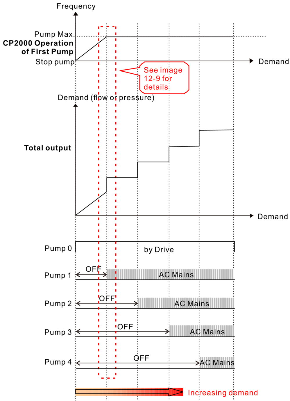
图 12-8 定量控制动作时序 - 增加需求
