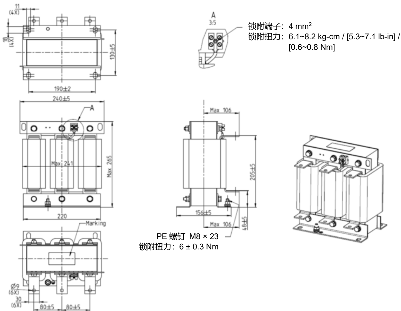
图 7-18 单位: mm
