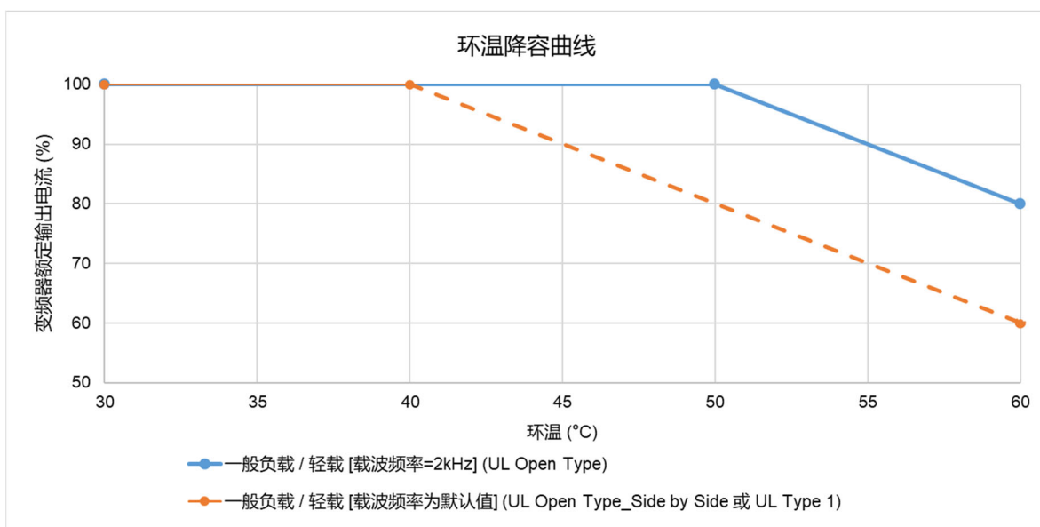
环境温度-降容曲线图
