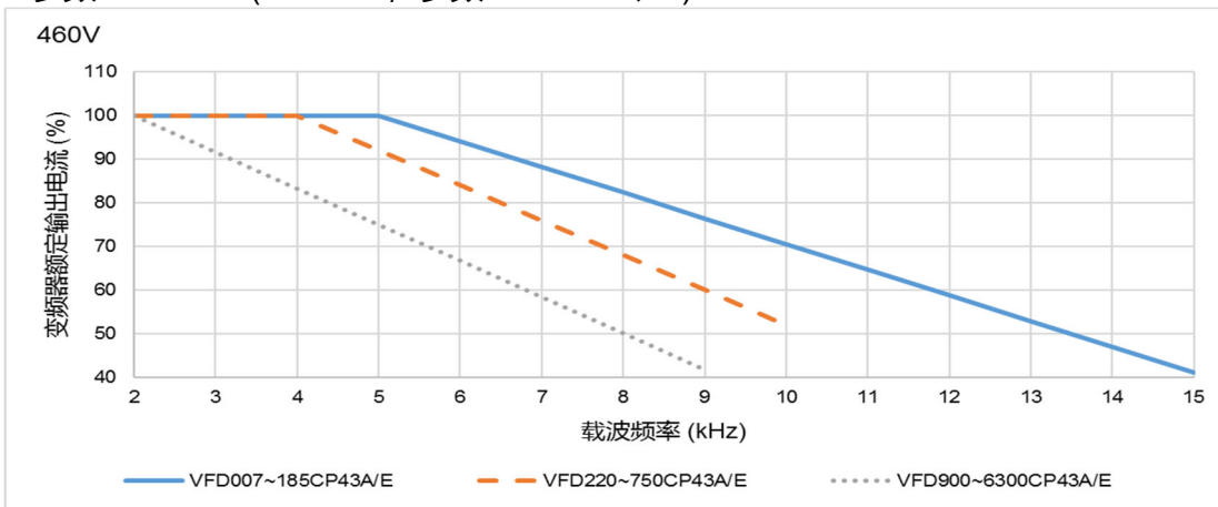
进阶控制模式下 460V 机种于不同载波下之输出电流降容额定 (单位: %)
