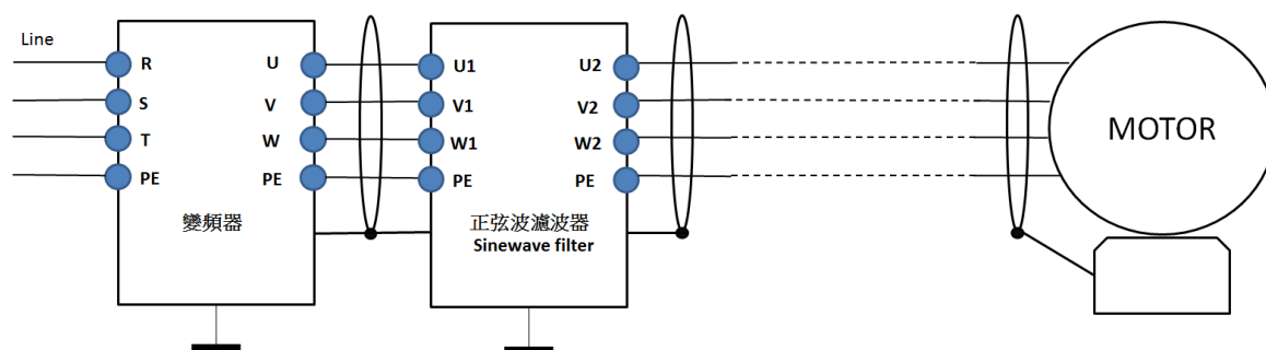
图 7-39 屏蔽线接线示意图
