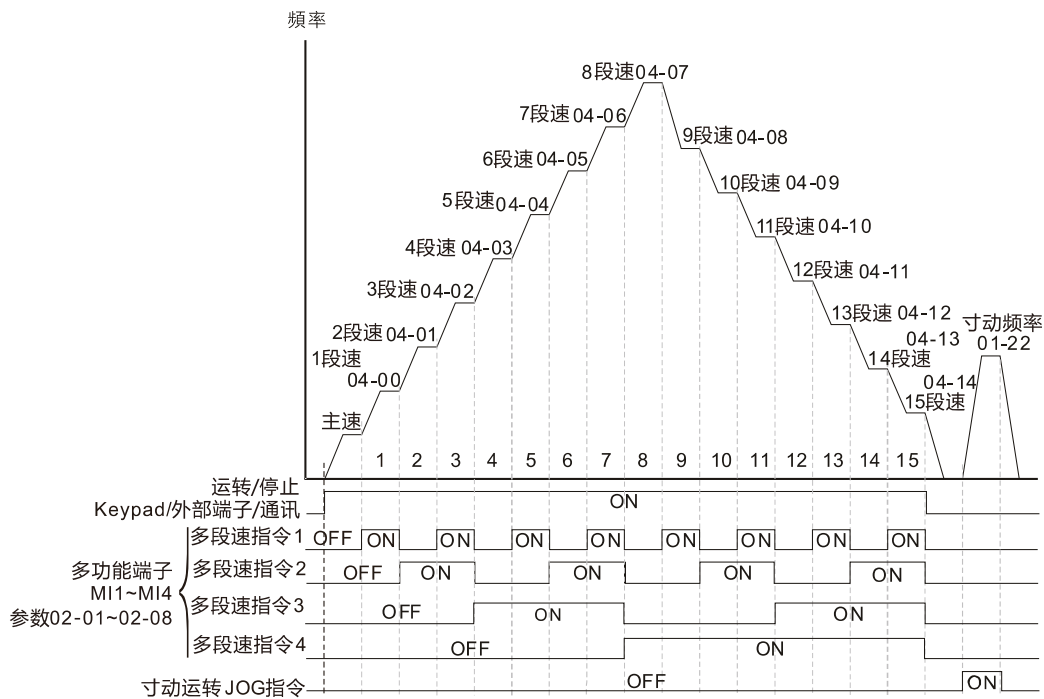
多段速与外部端子动作时序图
