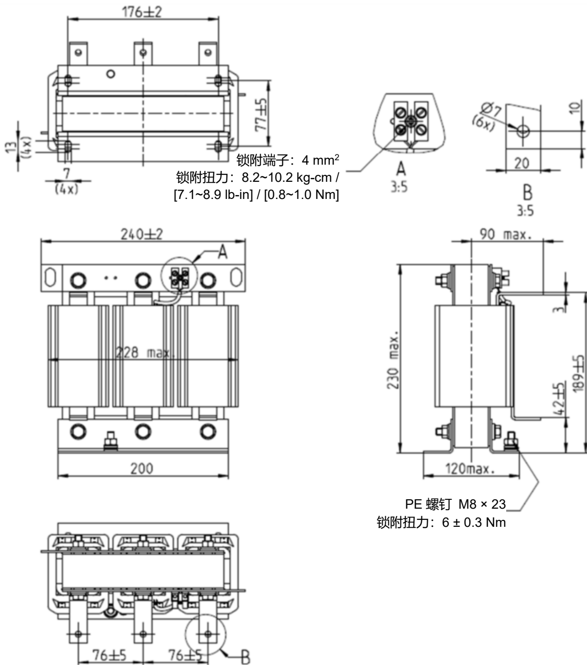
图 7-14 单位: mm
