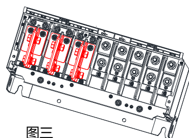
Copper Assy. 安装完成示意图
