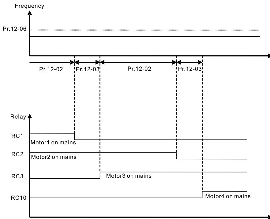
图 12-14 于定量控制平衡下执行定时循环
