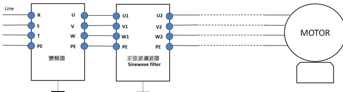
图 7-38 非屏蔽线接线示意图
