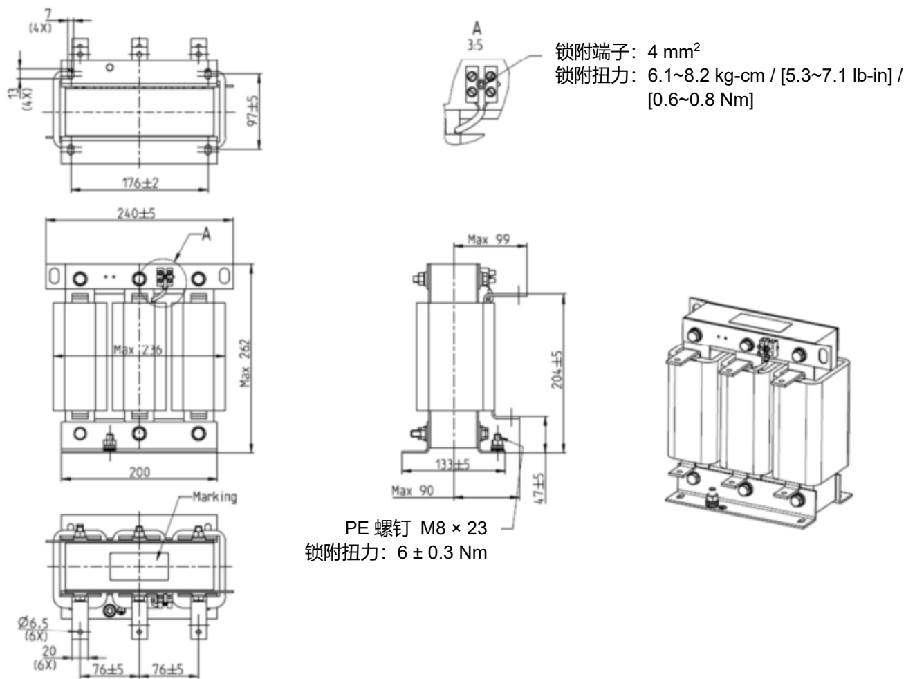
图 7-16 单位: mm
