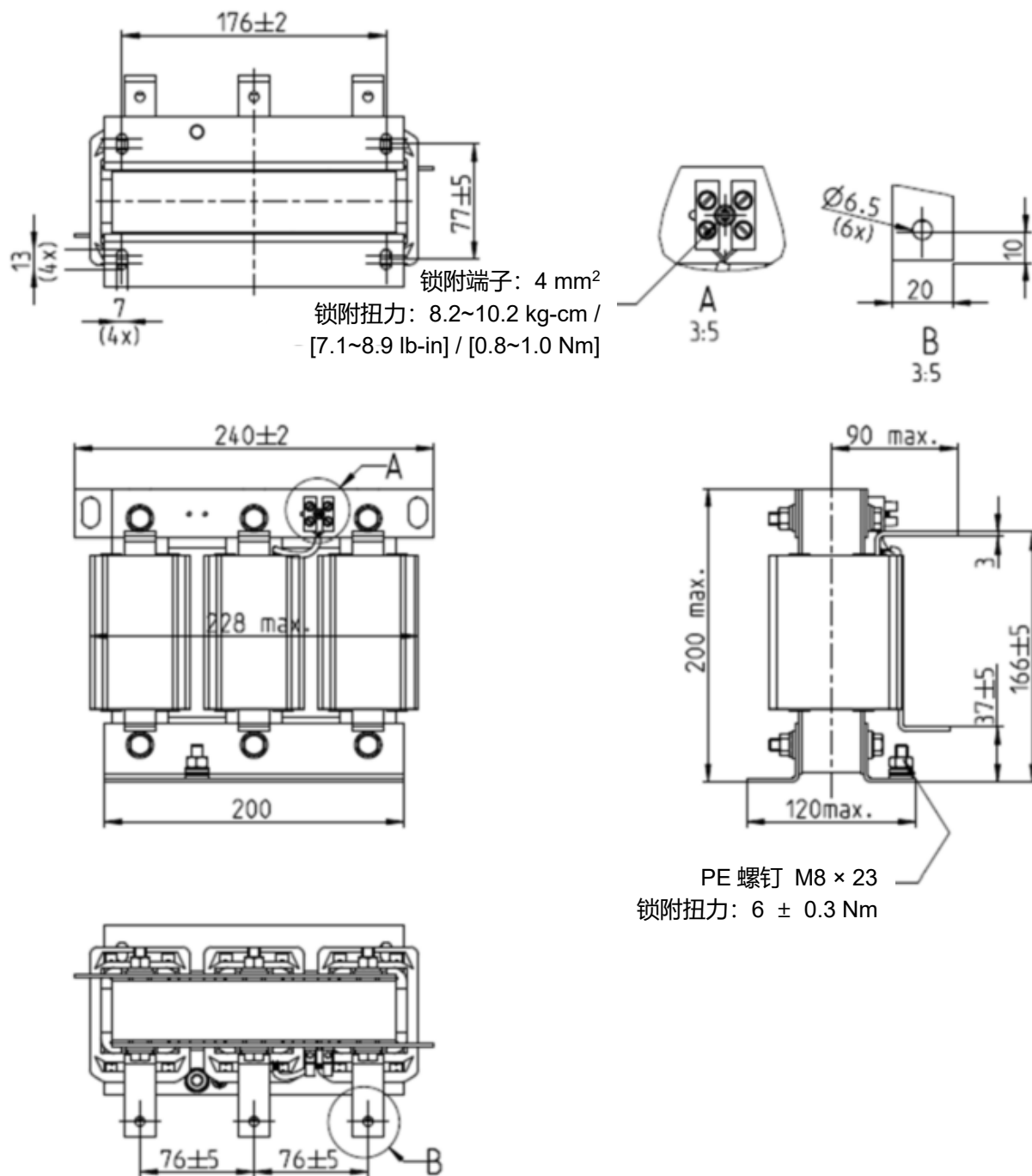
图 7-12 单位: mm
