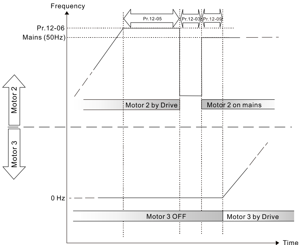
图 12-15 定量循环输出延迟切换时序
