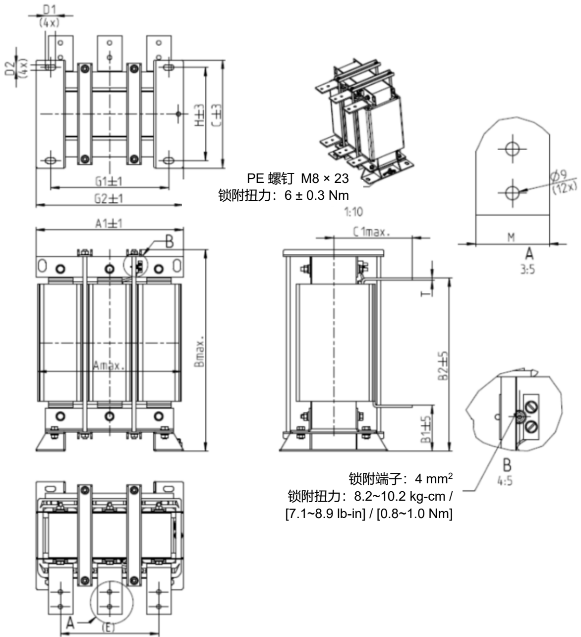
图 7-25 单位: mm
